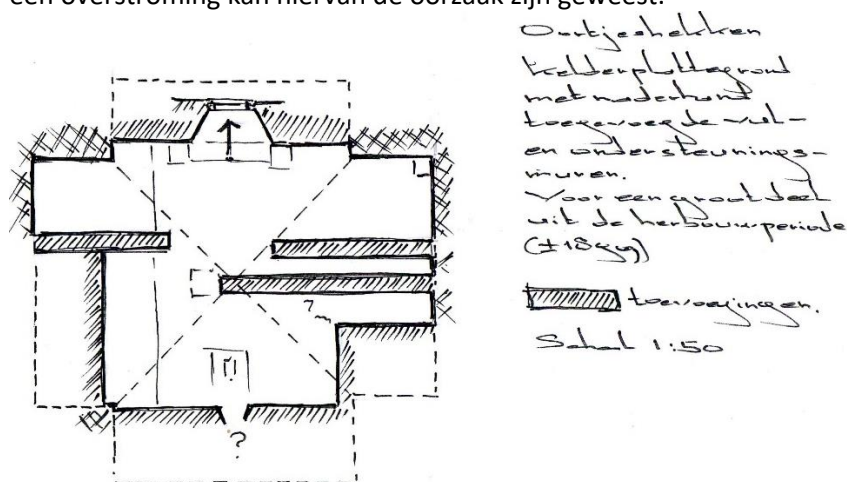
Plattegrond van de kelder met de later toegevoegde vul- en ondersteuningsmuren (gearceerd)
