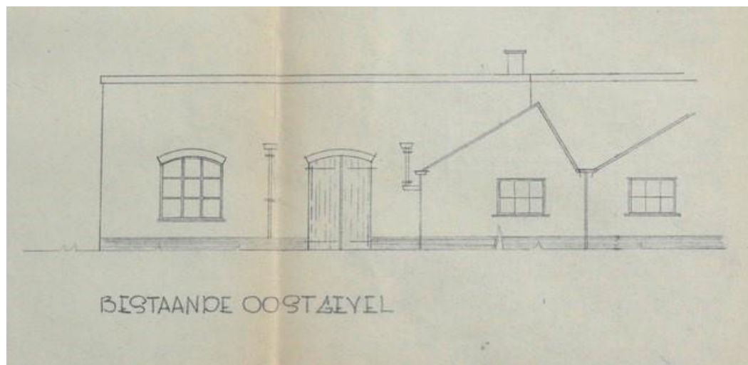
Bouwtekening voor de uitbreiding van 1960
