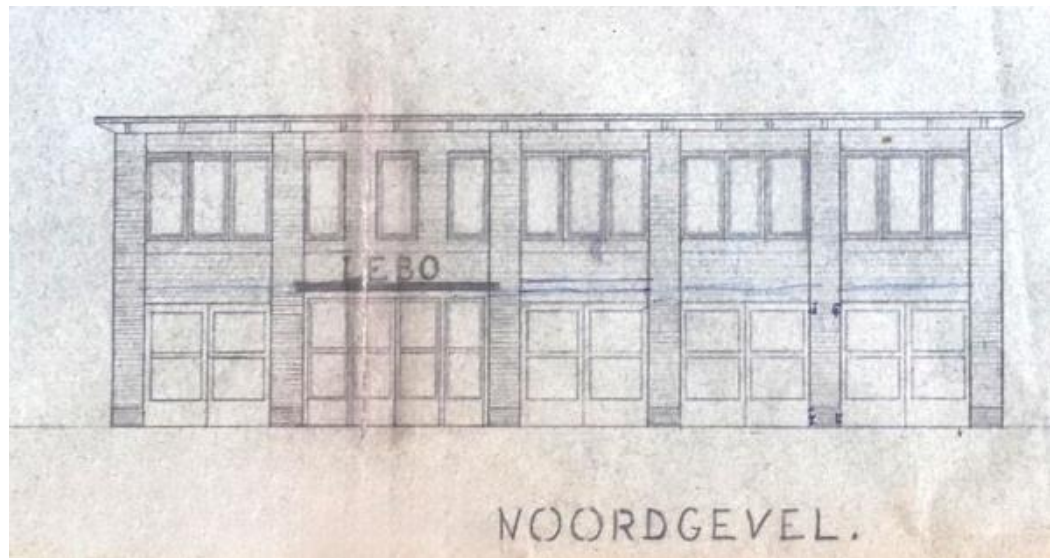
Bouwtekening voor de uitbreiding van 1954
